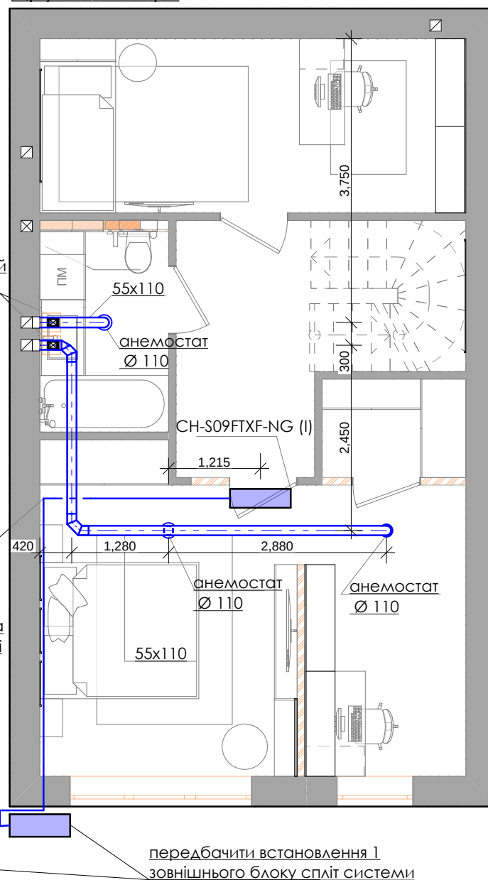
Схема вентиляції
